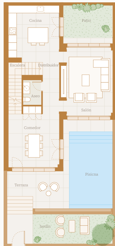
PLANTA BAJA
